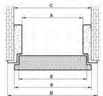
Ościeżnica drzwi
