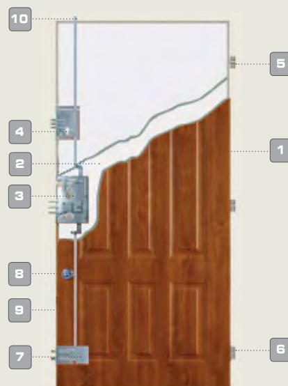
GRUBOŚĆ SKRZYDŁA 57 mm
