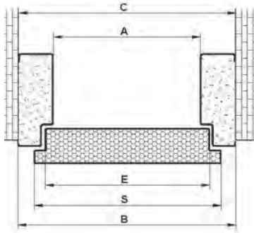
Ościeżnica drzwi
