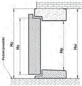
Ościeżnica drzwi, próg
