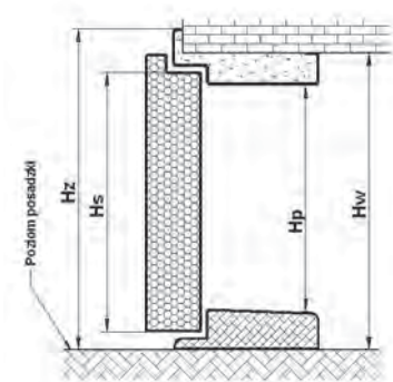
Ościeżnica drzwi, próg
