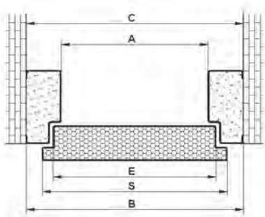
Ościeznica drzwi
