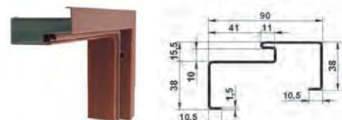
OŚCIEŻNICA ASYMETRYCZNA Z USZCZELKĄ FA (do drzwi TT PLUS, TT MAX, GTT PLUS, GTT MAX)
