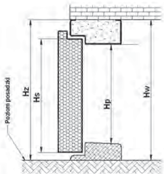
Ościeznica drzwi, próg
