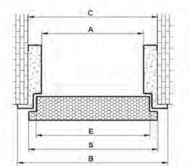
Ościeżnica drzwi
