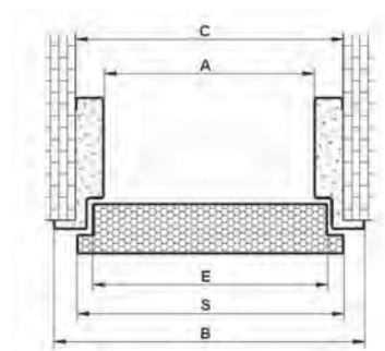
Ościeżnica drzwi
