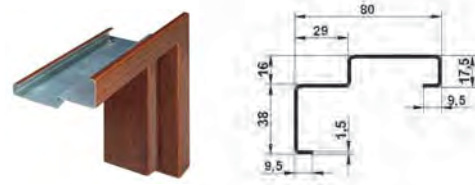
OŚCIEŻNICA NAROŻNIKOWA BEZ USZCZELKI FN (do drzwi TT i GTT)
