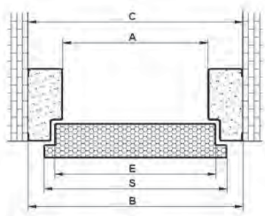
Ościeżnica drzwi
