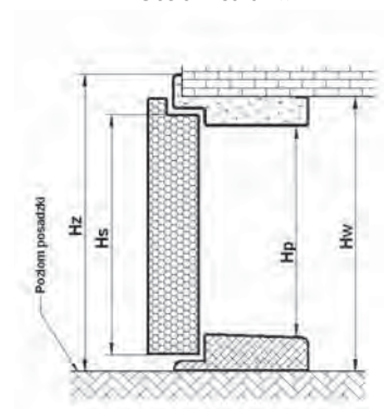
Ościeżnica drzwi, próg
